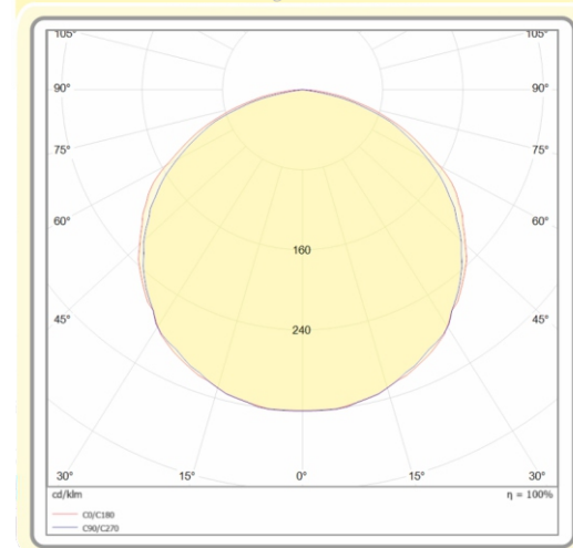
Diagramma polare EKOMINI32 Polar diagram EKOMINI32
