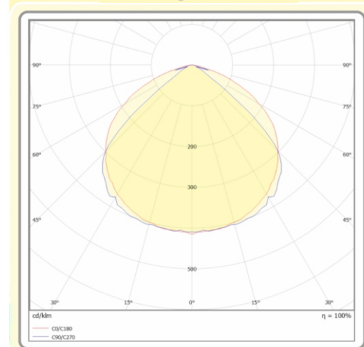
Diagramma polare NICE EKO Polar diagram NICE EKO
